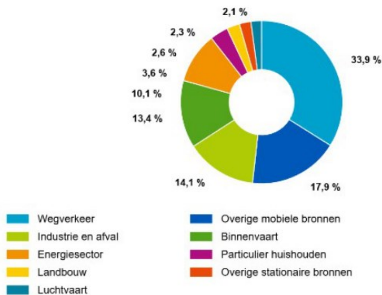
Emissie van stikstofoxiden (NO x ) naar bron, 2022
